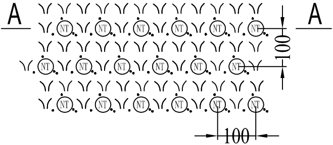
场地绿化典型设计平面图 1:100
