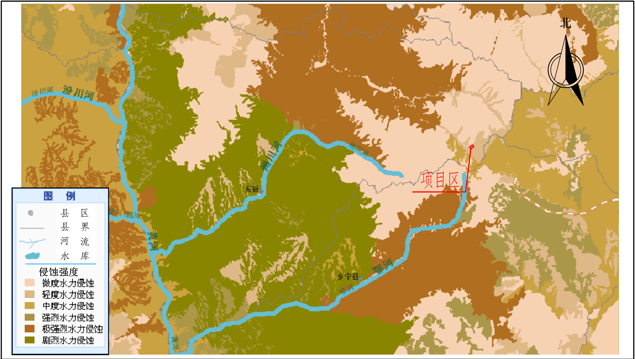
附图5 项目区土壤侵蚀强度分布图
