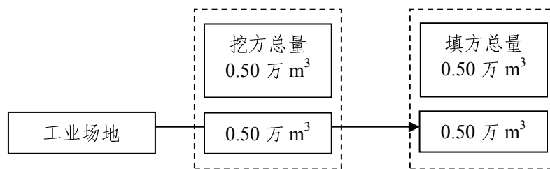
图 2-1 总土石方平衡流向框图
